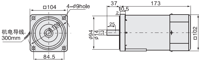
結構：電動機 重量：5kg
