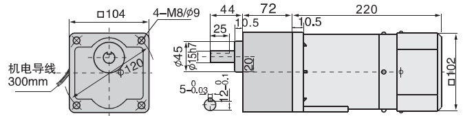
結構：減速器+電動機+剎車器 重量：7.1kg
