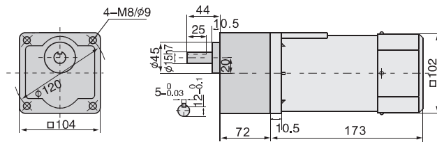
結構：減速器+電動機 重量：6.7kg
